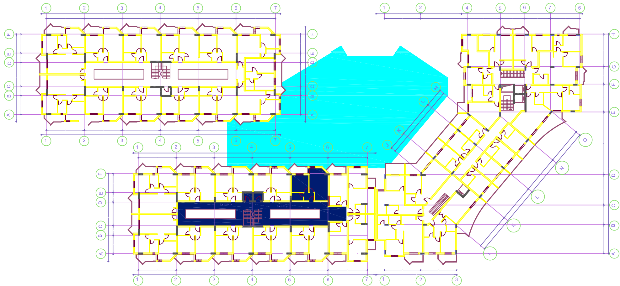
PLANIMETRIA E APARTAMENTIT 5 / KT DYTE SH 1: 100 ( OBJEKTI 2 )
