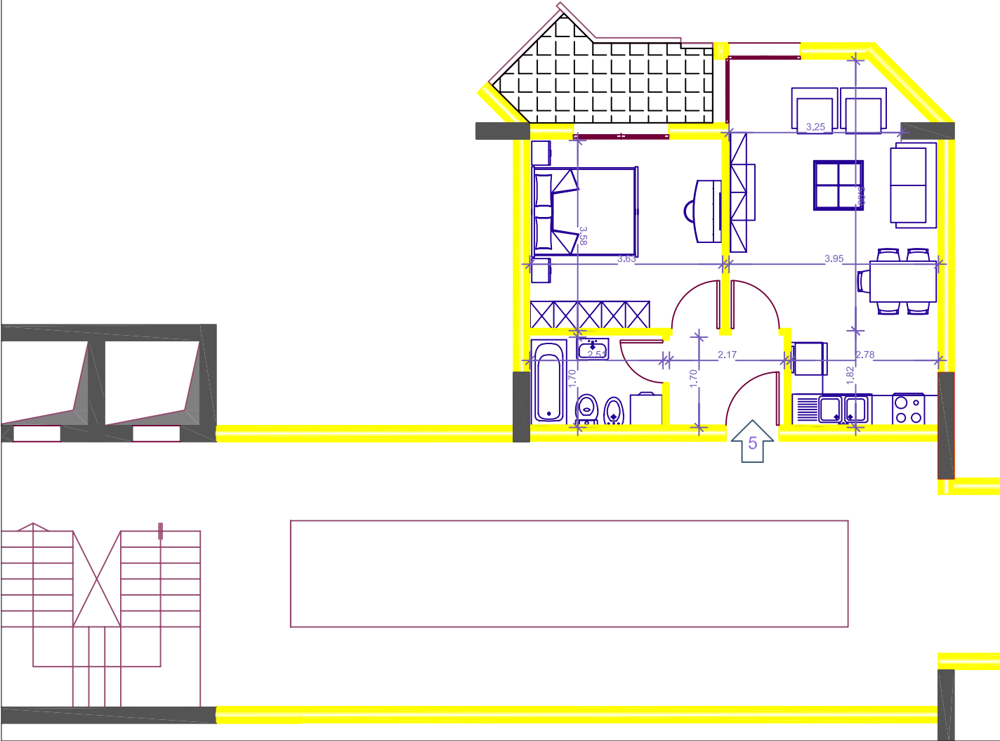
PLANIMETRIA E APARTAMENTIT 5 / KT DYTE SH 1: 100 ( OBJEKTI 2 )
