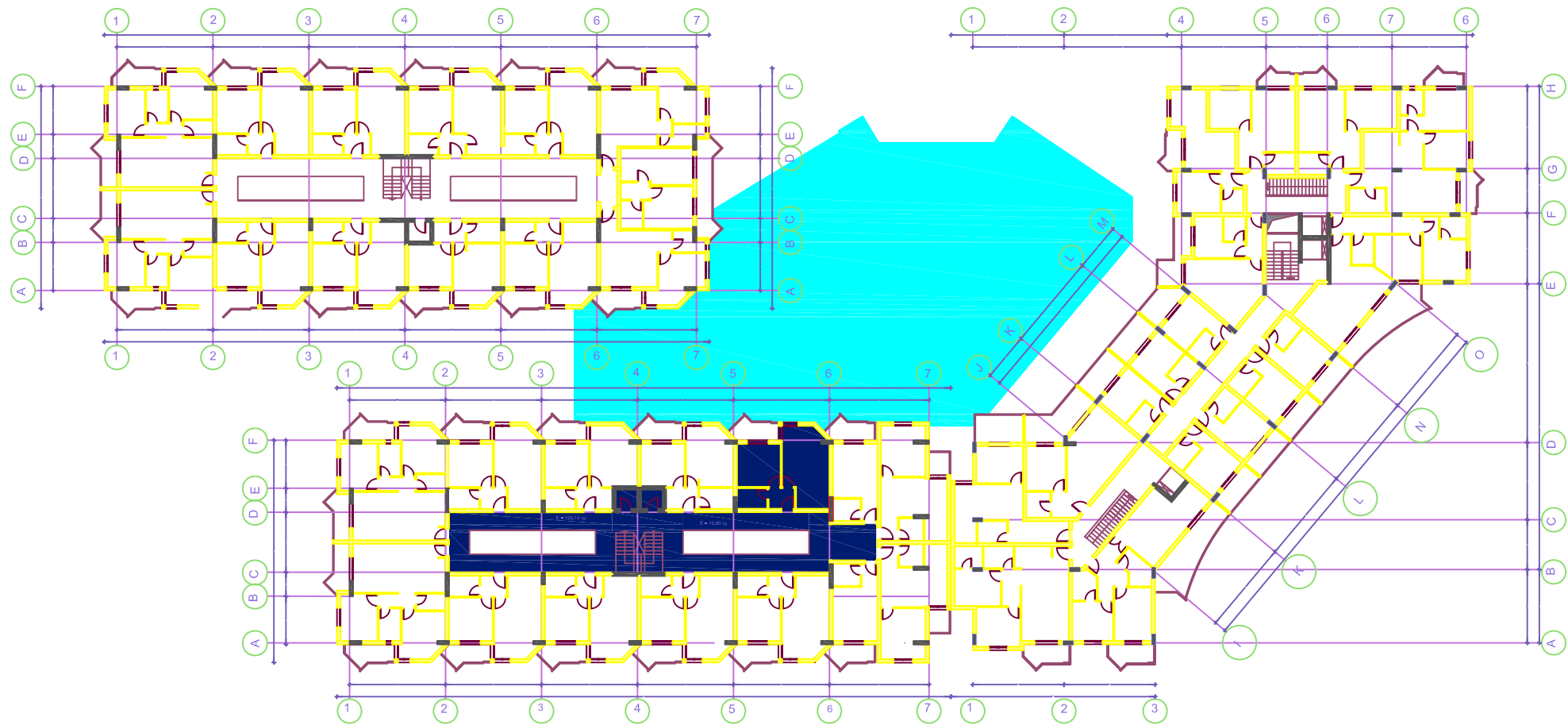
PLANIMETRIA E APARTAMENTIT 5 / KT PESTE SH 1: 100 ( OBJEKTI 2 )
