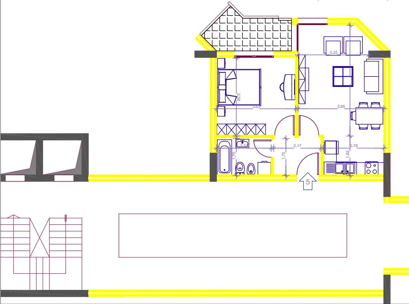
PLANIMETRIA E APARTAMENTIT 5 / KT PESTE SH 1: 100 ( OBJEKTI 2 )
